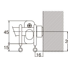
正面図
