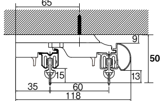
天井付ダブルブラケット付 (ブラケット幅=21mm)
