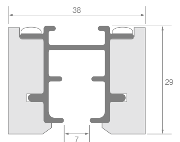
レール断面図 (単位: mm)
