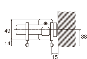
正面図
