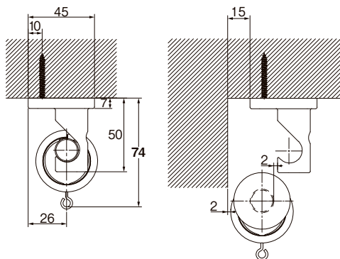
天井付シングルブラケット付 (ブラケット幅=20mm)
