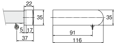
メタルキャップストップM(ダブル) (正面図) (側面図)
