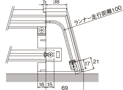
(下面図)
