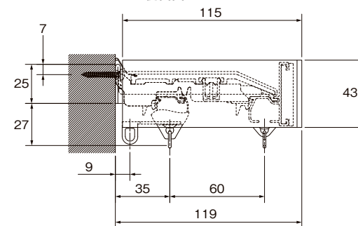
カバートップII MC セット側面図
