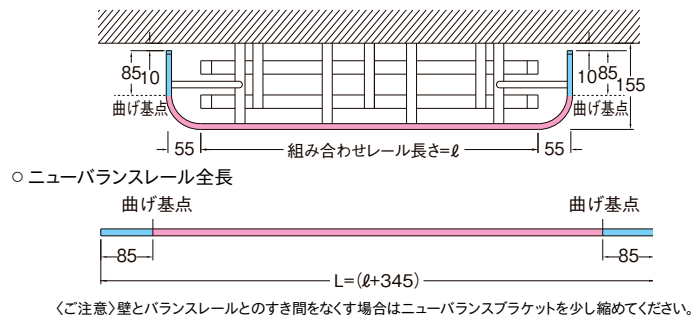
基本取付図
