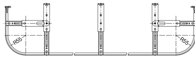
基本取付図
