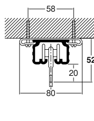
天井付シングルブラケット付 (ブラケット幅=38mm) (ランナー使用)
