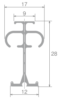
レール断面図 (単位: mm)
