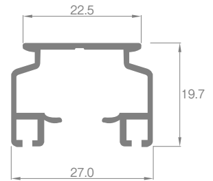
レール断面図 (単位: mm)
