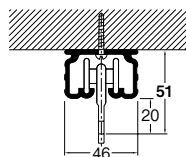
天井直付 (ランナー使用)
