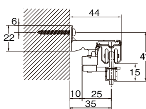
カバートップIIセット平面図
