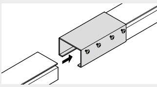
大型レールをカバージョイントに差し込みます。
