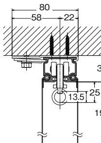
天井シングルブラケット付 (ランナー)
