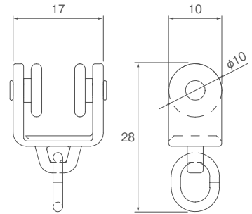
ランナー寸法図 (単位: mm)
