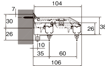
カバートップIIセット側面図
