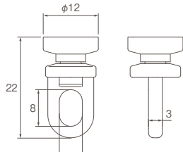
ランナー寸法図 (単位: mm)
