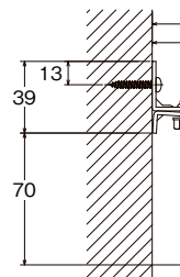
シングルブラケット付 (カラビナランナー)
