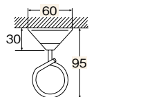
点滴フック寸法図（単位：mm）
