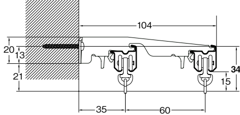
NTダブルブラケット付 (ブラケット幅=44mm)
