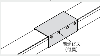
付属の4本の固定ビスを締めるとレールが固定されます。
