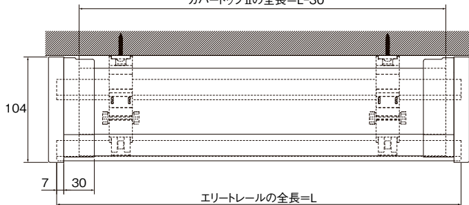
カバートップIIセット平面図
