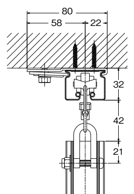
天井シングルブラケット付 (特殊ランナー+ 間仕切サイドポール+U継金具) (間仕切中間ポール+U継金具)
