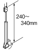
テンションプーリー 240
