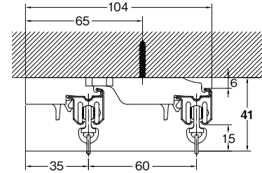
天井付ダブルブラケットII付 (ブラケット幅=21mm)
