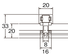
天面図
