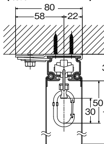
天井シングルブラケット付 (カラビナランナー-S) (特殊カラビナランナー)
