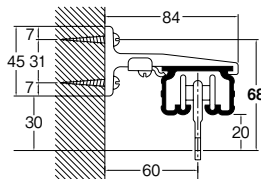
シングルブラケット付 (ブラケット幅=34mm) (ランナー使用)
