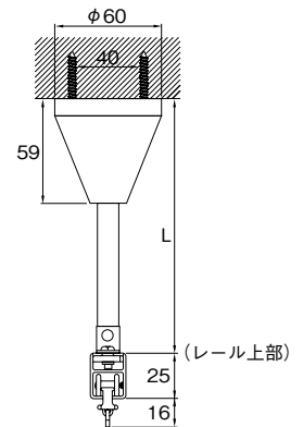
固定吊棒セット
