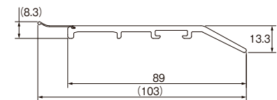
カバートップII本体側面図
