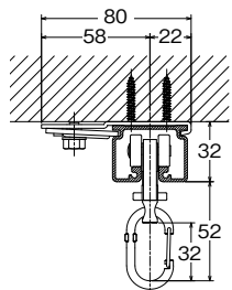
天井シングルブラケット付 (カラビナランナー)
