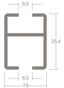
レール断面図 (単位: mm)
