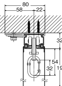
天井シングルブラケット付 (カラビナランナー)
