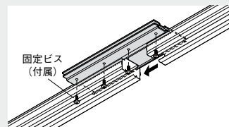
固定ビス(付属)レールをはさみ込み固定ビスを締めるとレールが固定されます。
