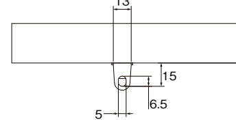
共通後入れ中間ストップ (ストップ幅=13mm)
