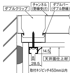
軽量鉄骨下地 天井後付 10kg
