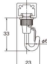
T/TCワンタッチフック 30B
