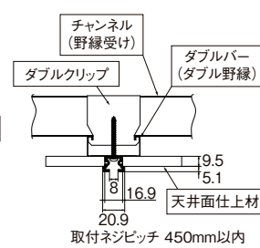
軽量鉄骨下地 天井先付(両ツバ仕様) 10kg
