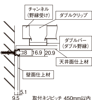
コンクリート下地 正面先付(片ツバ仕様) 30kg
