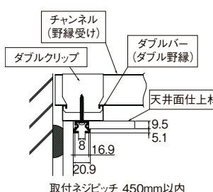
軽量鉄骨下地 天井先付(片ツバ仕様) 10kg
