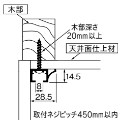
木下地 天井後付 30kg
