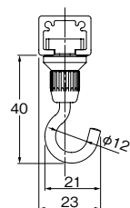
T/TCフック 30H
