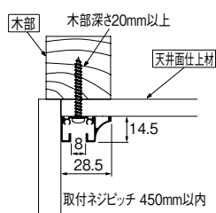
木下地 天井後付 15kg
