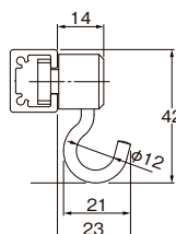
ランナーフック 30A(ランナーフックA)
