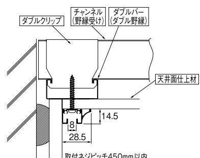
軽量鉄骨下地 天井後付 10kg
