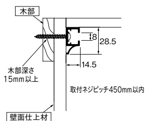
木下地 正面後付 30kg
