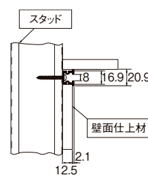
軽量鉄骨下地 正面先付(片ツバ仕様) 10kg
