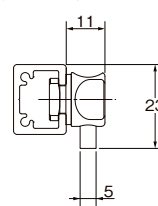
T/TCワンタッチフック 30B
