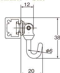
T/TCワンタッチフック 30A
