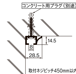
コンクリート下地 天井後付 30kg
