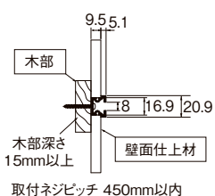
木下地 正面先付(両ツバ仕様) 30kg
