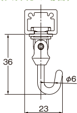
ランナーフック 30B(ランナーフックB)
