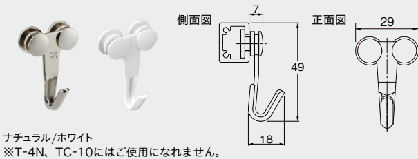
T ランナーフック 30B(ランナーフックB)(正面付)
