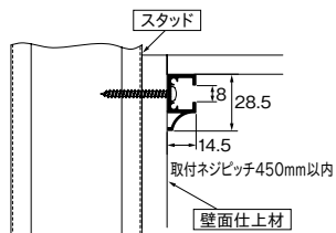
軽量鉄骨下地 正面後付 10kg
