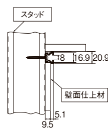
軽量鉄骨下地 正面先付(片ツバ仕様) 10kg
