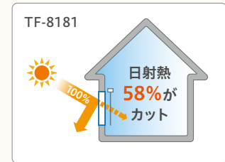
TF-8181 パーチカルブラインドを付けた場合 複層ガラス窓 + パーチカルブラインド \eta = 0.42 (TF-8181)
